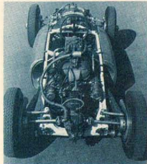
Cisitalia 360 da Gran Premio. Si tratta dell'unico esemplare che sia stato completato e che abbia funzionato. Nel 1949 venne spedita in Argentina, nel 1960 venne riportata in Europa e messa nel museo della Porsche a Stoccarda. Le foto sono state scattate alla Porsche. Un secondo esemplare (non funzionante) si trova nel museo di Tom Wheatcroft nella Donington Collection.
